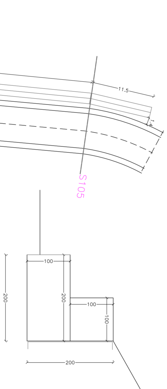
DISEGNI ESECUTIVI SCALA 1:50
