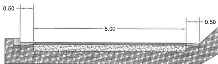
SEZIONE TIPO - KM 5+000
