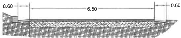
SEZIONE TIPO - KM 4+600
