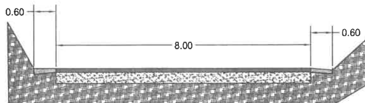
SEZIONE TIPO - KM 2+200
