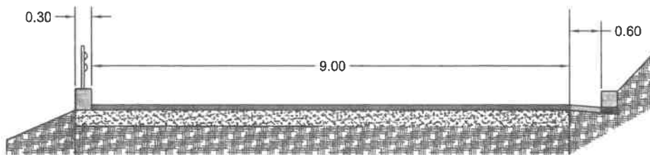
SEZIONE TIPO - KM 2+000
