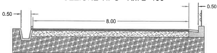
SEZIONE TIPO - KM 2+400
