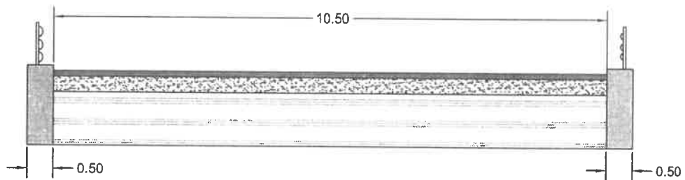
SEZIONE TIPO - KM 1+000 VIADOTTO GIANGUZZO
