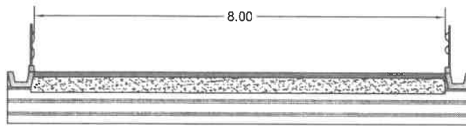
SEZIONE TIPO - KM 13+300 VIADOTTO
