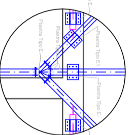
Plastrina tipo E, P max = 1834 kg
