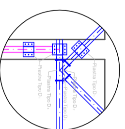
Plastrina tipo D, P max = 1637 kg
