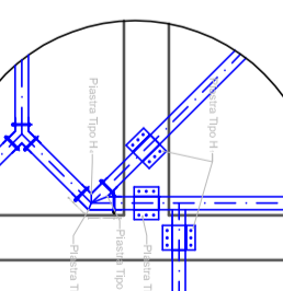
Plastrina tipo H, P max = 1637 kg
