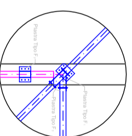
Plastrina tipo F, P max = 2511 kg
